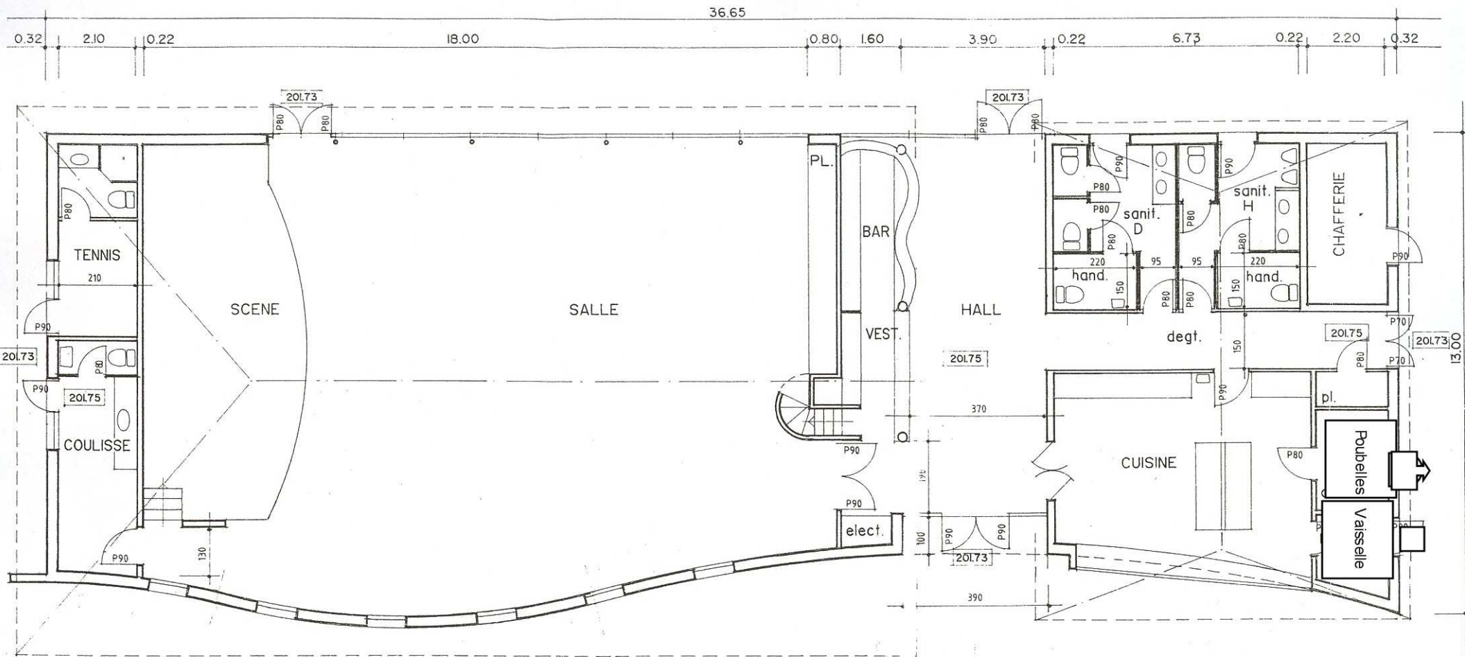
Plan de masse salle des fêtes
